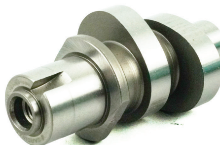
NAME : RACING CAM HIGH LIFT CODE : CR1VPHL COLOUR : - MODEL : SRL115 FI NOTE : IN:3.4 / EX:3.3 XXNPXX
